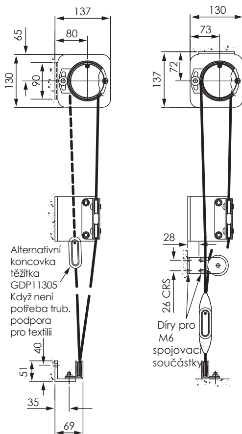
Pohled A-A
